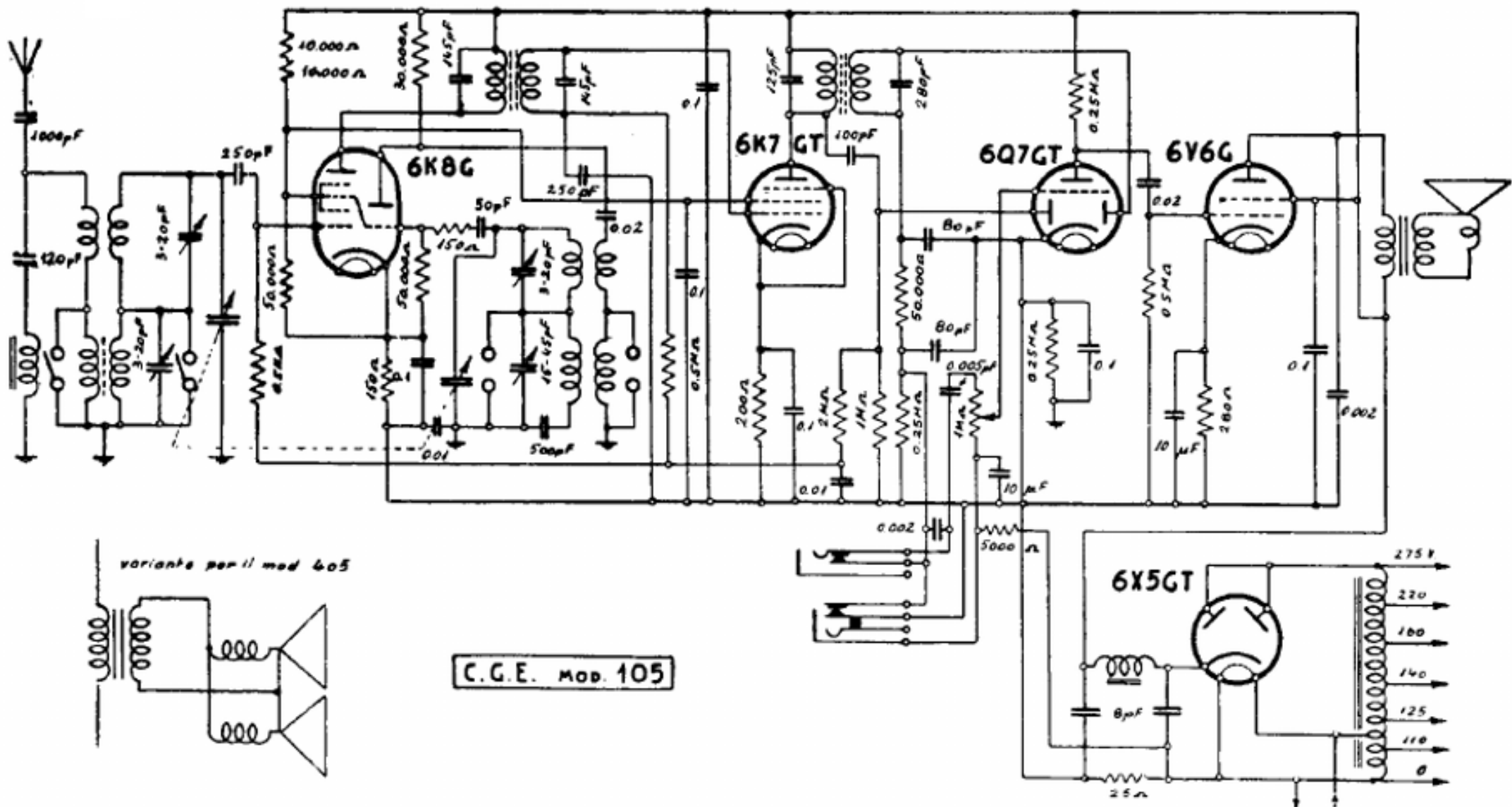
COMPAGNIA GENERALE DI ELETTRICITÀ. — Modelli « 105 » e « 405 ». — Produzione 1939-1940. — Media frequenza: 468 kHz.
